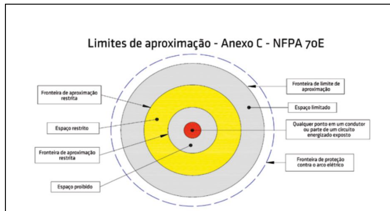
Figura 9 - Limite de Aproximação para Riscos Elétricos
